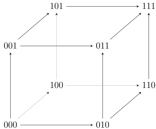
Рис. 11.6. Булев куб
